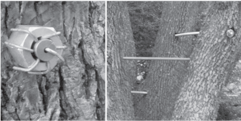
Укрепление дерева стяжками
